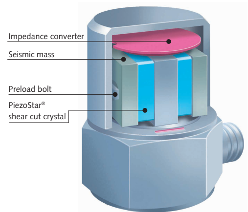
PiezoStar® IEPE shear accelerometer
